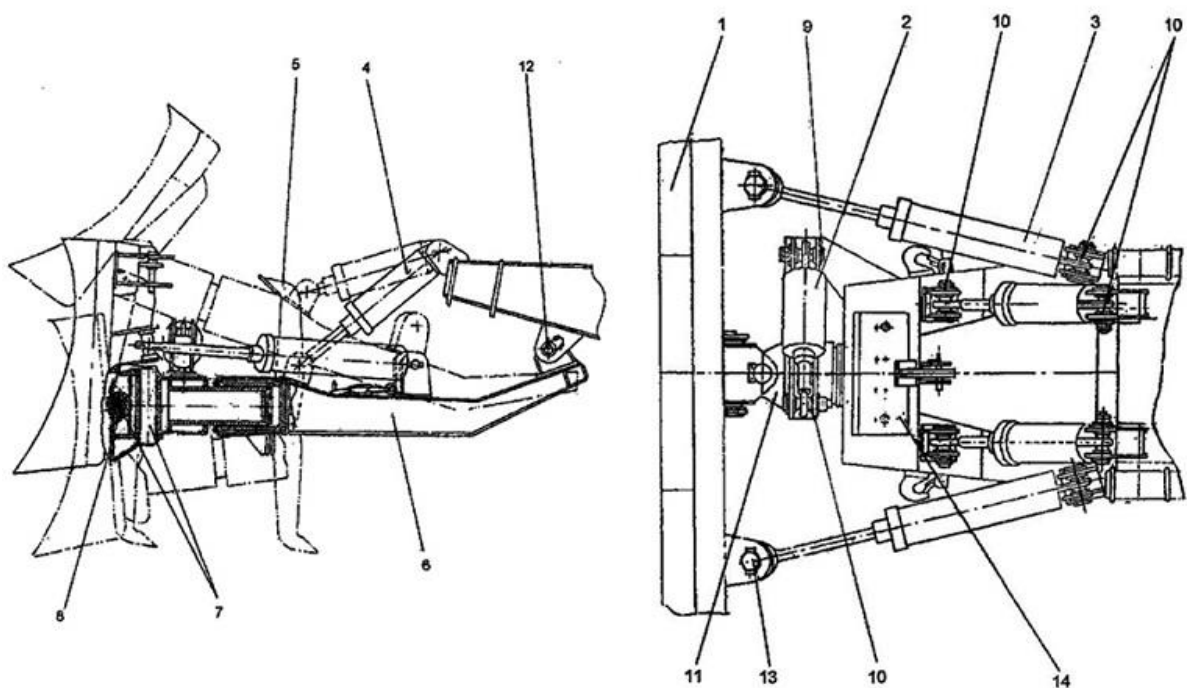
Оборудование бульдозерное БКУ.00.00.000
